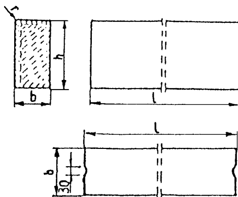
Rys. 1. Wymiarowanie krawężników
