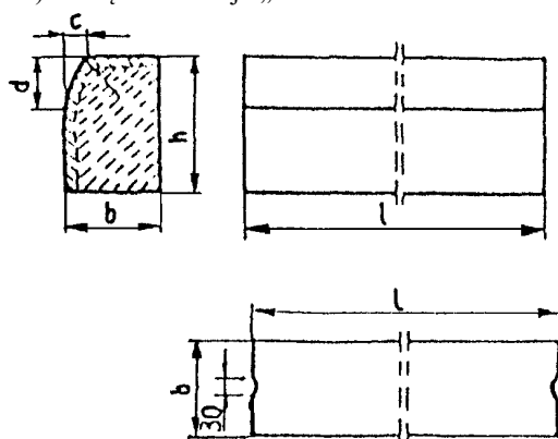
a) krawężnik rodzaju „a”
