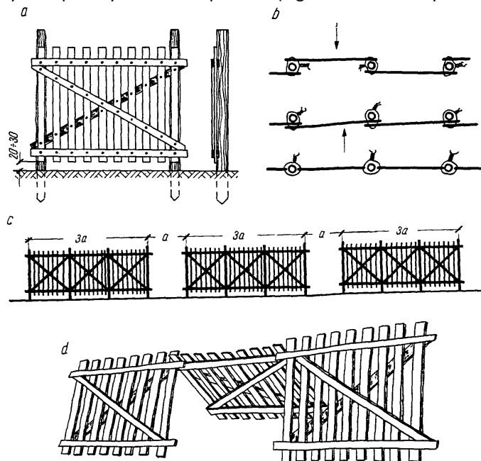
Rys. 4. Sposoby ustawiania płotków (wg K. Sokalski: Utrzymanie dróg, WKiŁ, 1964)
