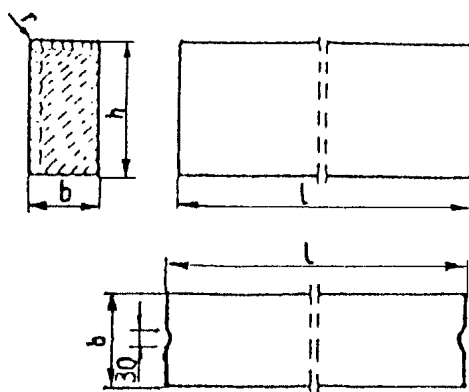
Rys. 1. Wymiarowanie krawężników
