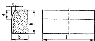
a) krawężnik rodzaju „a”
