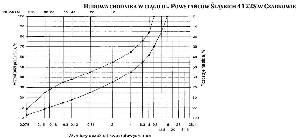
Rys. 10. Krzywe graniczne uziarnienia mieszanki mineralnej BA od 0 do 12,8 mm do warstwy wiążącej, wyrównawczej i wzmacniającej nawierzchni drogi o obciążeniu ruchem KR1 lub KR2
