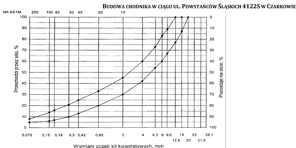
Rys. 13. Krzywe graniczne uziarnienia mieszanki mineralnej BA od 0 do 16 mm do warstwy wyrównawczej nawierzchni drogi o obciążeniu ruchem od KR3 do KR6
